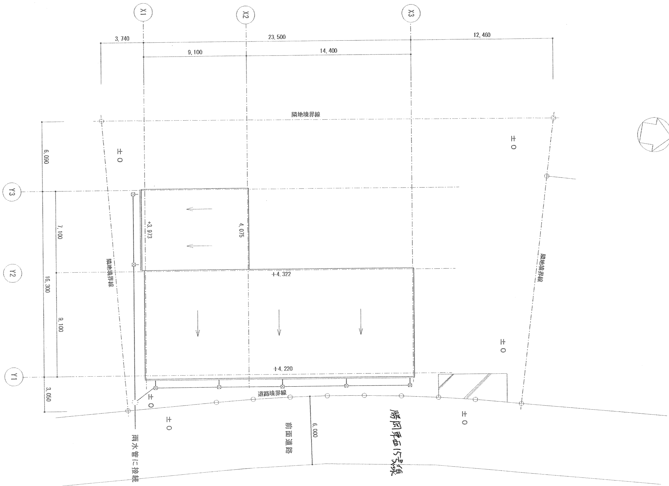
配置図 S=1/200
